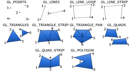
Şekil 1. İlkel (Primitif) Geometrik Nesnelere
