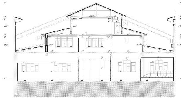
B-B KESİTİ Ö: 1/50
