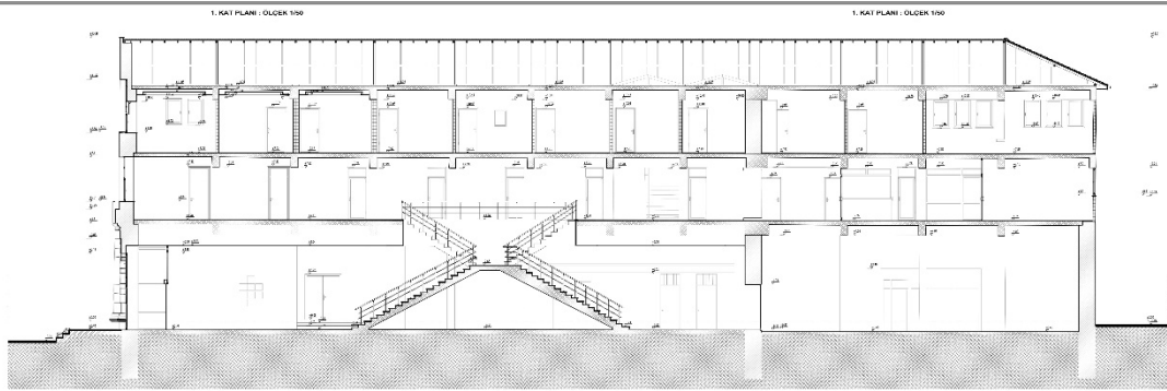
A-A KESİTİ Ö: 1/50
