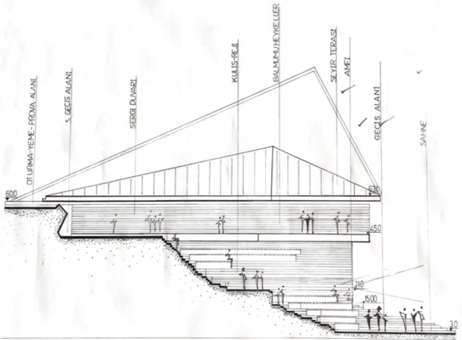
A-A KESİTİ
